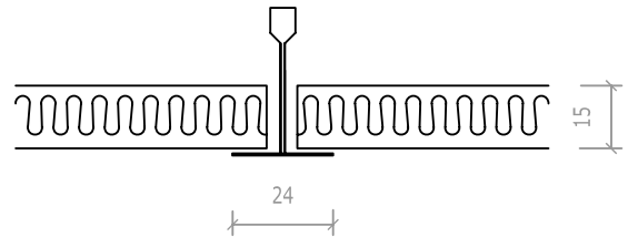
T24 Square Edge Scale 1:2
