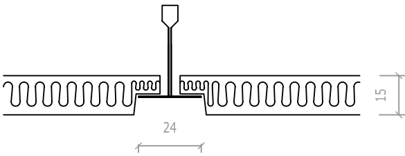
T24 Reveal Edge Scale 1:2
