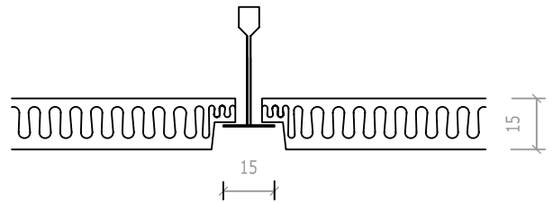
T15 Reveal Edge Scale 1:2
